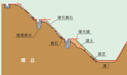
前方部復元計画模式図
