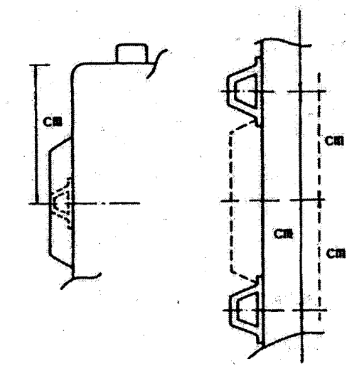
防舷材測定位置図
