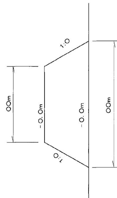
標準断面図
