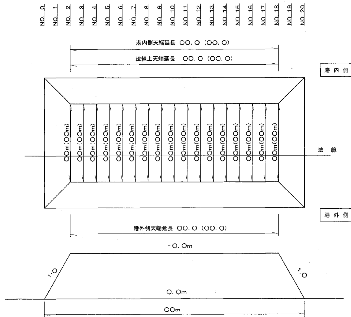
敷砂 平面図
