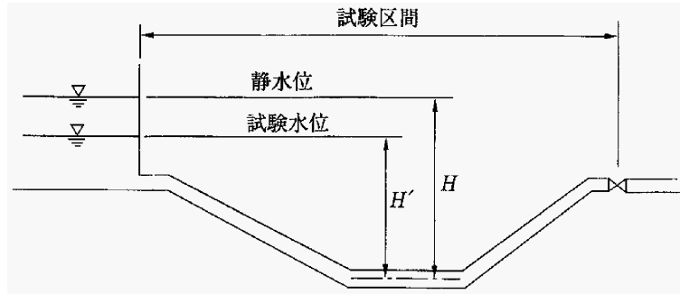
図-1 試験水頭のとり方
