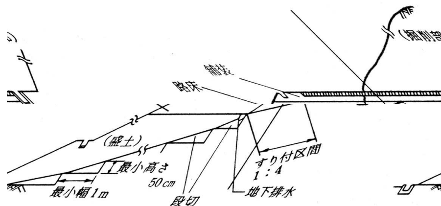
図2-2 盛土基礎地盤の段切
