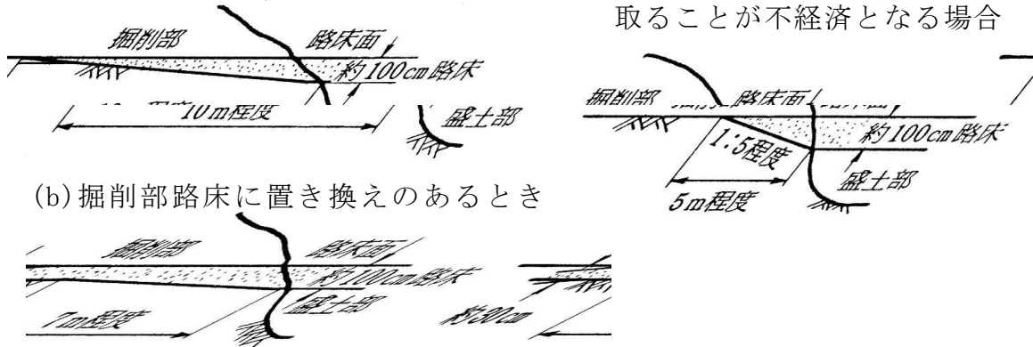
図2-3 掘削（切土）部、盛土部接続部のすり付け
