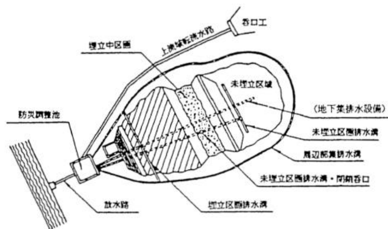
雨水集排水設備の概念図
