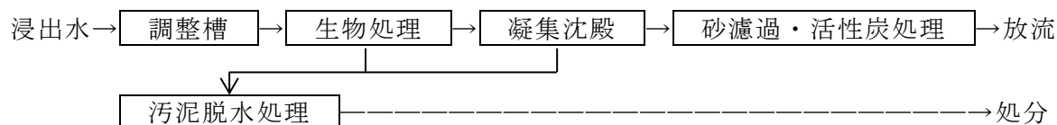
浸出水の処理フロー
