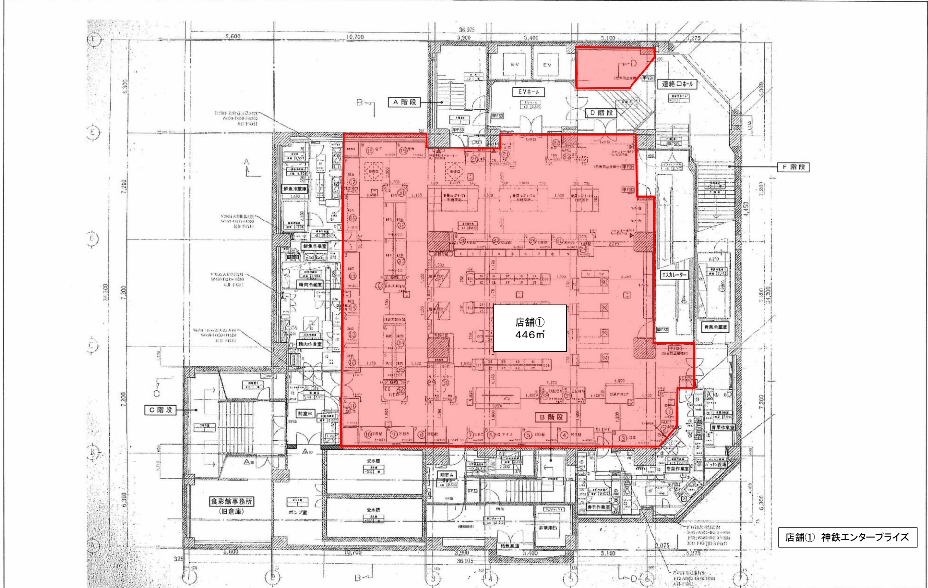
地下2階平面図
