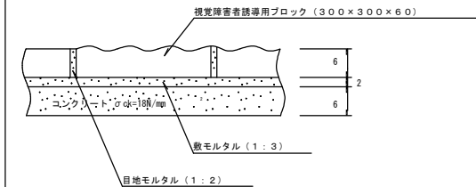
視覚障害者誘導用ブロック工 (300×300×60)
