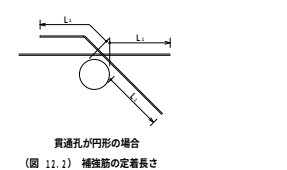
(図 12.2) 補強筋の定着長さ
