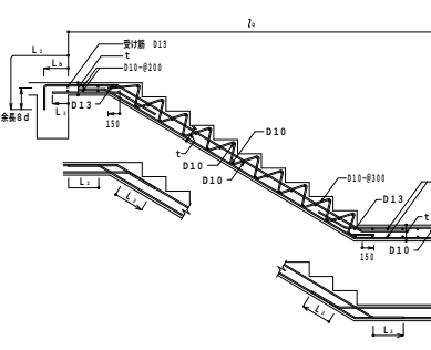
(図 11.2) 二辺固定スラブリ筋階段配筋 (その1)
