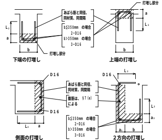
(図 13.1) 梁の打増し補強配筋
