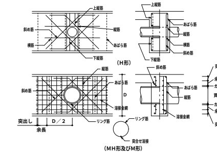
(図 12.1) 梁貫通孔補強筋の名称等
