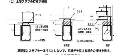
(図 10.9) 打継ぎ補強配筋
