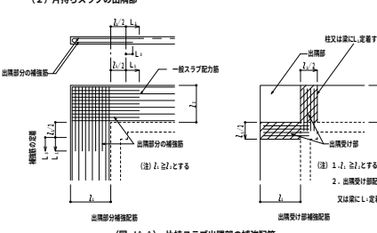
(図 10.8) 片持ちスラブリ筋の出隅部の補強配筋
