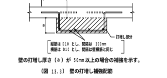
(図 13.3) 壁の打増し補強配筋
