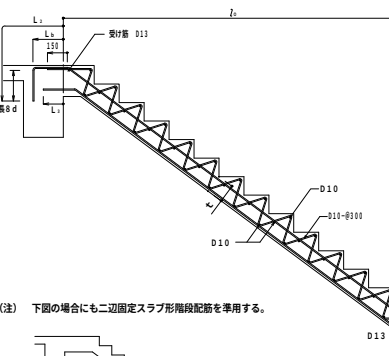
(図 11.2) 二辺固定スラブリ筋階段配筋 (その1)
