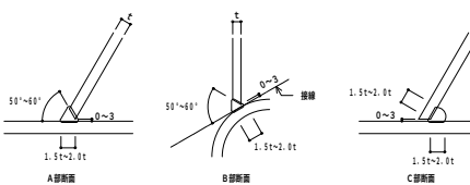
図 2.15 鋼管分岐継手詳細（単位：mm）
