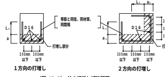
(図 13.2) 柱の打増し補強配筋
