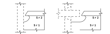
図 2.11 改良型スカラップ（柱梁接合部）
