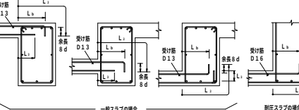
(図 10.3) スラブリ筋の定着長さ及び受け筋 (その2)
