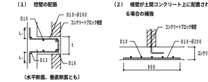
(図 12.4) 壁付き土間コンクリートの補強
