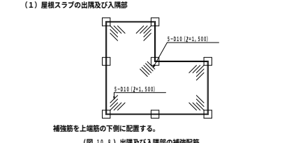
(図 10.7) 出隅部及び入隅部の補強配筋
