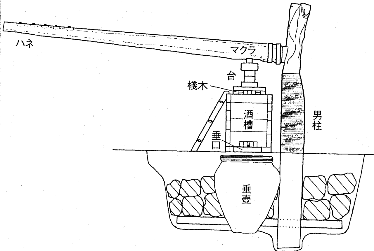
男柱遺構復元図(伊丹市『旧岡田家住宅保存修理工事報告書』より)
