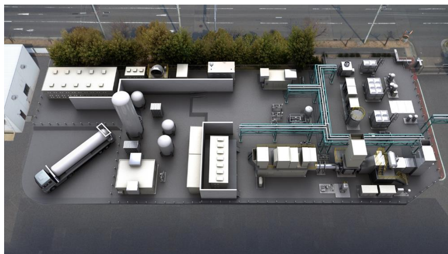
図2 水素コージェネレーションシステムのプラントの俯瞰図(CG)
