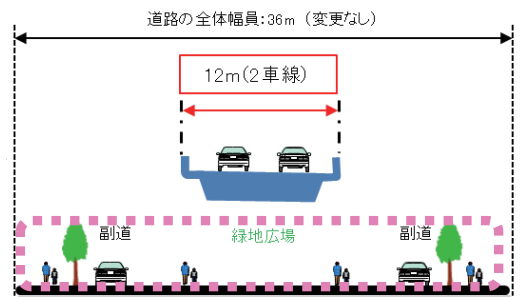
①-①断面 イメージ図【変更後】
